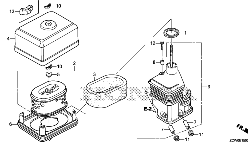
MUFFLER
