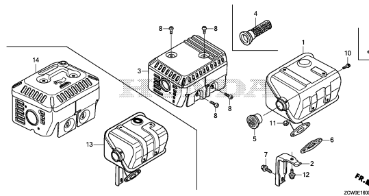
MUFFLER
